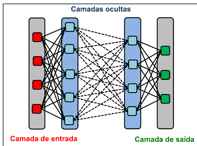
Figura 2. Representação do algoritmo de aprendizado profundo.
